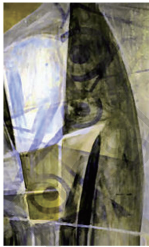
高光谱伪彩色图像
